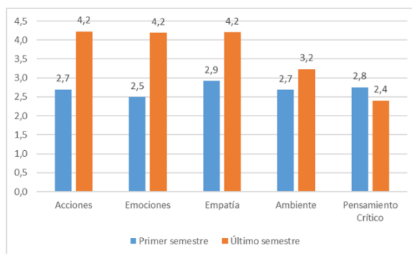
Figura 6. Comparación de medias de estadísticos en las variables. Elaboración propia (2024)
