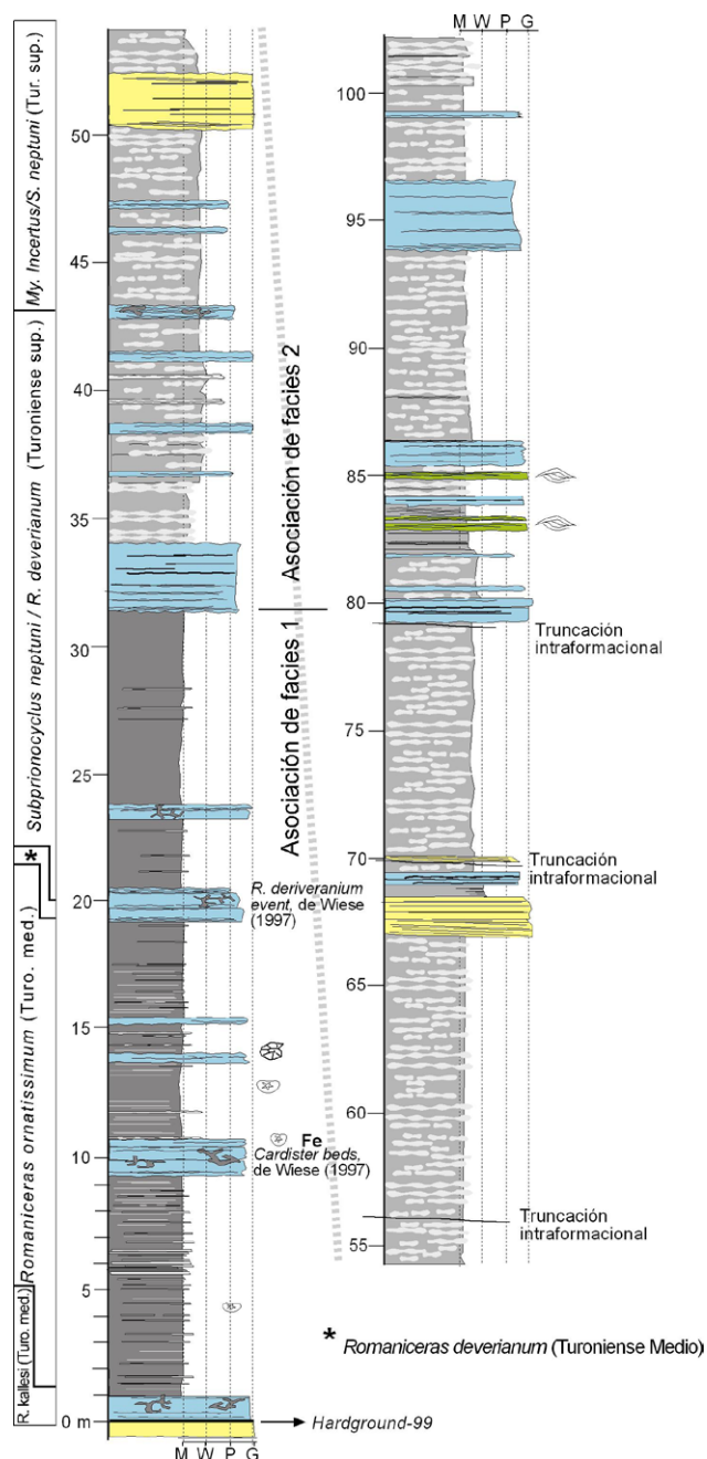
Fig. 4.- Columna estratigráfica de la Formación Sardinero en la sección de Portio, incluyendo distintos eventos y zonación bioestratigráfica de Wiese (1997). La sucesión continúa al menos 100 m con una monótona sucesión rítmica marga/caliza (ver Fig. 5).
