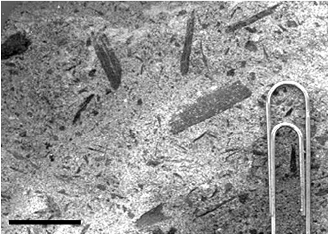
Figura 3. Restos vegetales carbonizados conservados entre lutitas arenosas en un bloque aloctóno en la Cantera Victoria-I, La Habana. Escala 1 cm. Carbonized vegetal remains preserved within sandy lutites in an alloctonous block at Cantera Victoria-I, La Habana. Scale 1 cm.
