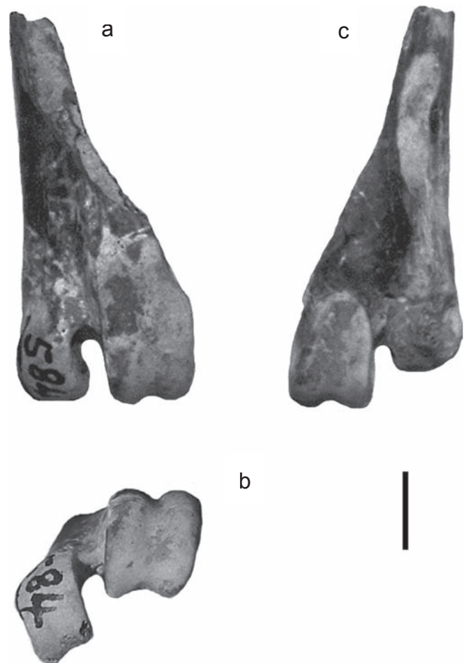
Figura 2. a-c, Ciconia maltha Miller, 1910, extremo distal de tarsometatarso izquierdo (MACN Pv 584) en vistas (a) anterior, (b) distal y (c) posterior. Escala 1 cm. Ciconia maltha Miller, 1910, distal extreme of left tarsometatarsus (MACN Pv 584) in (a) anterior, (b) distal, and (c) posterior views. Scale bar 1 cm.
