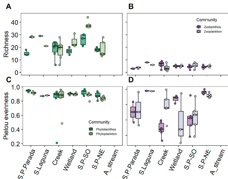
Figure 3. Richness (A, B) and Pielou evenness (C, D) of microalgae and invertebrate communities of Salar Pedernales Basin. Riqueza (A, B) y equitatividad de Pielou (C, D) de las comunidades de microalgas e invertebrados de la cuenca del Salar de Pedernales.
