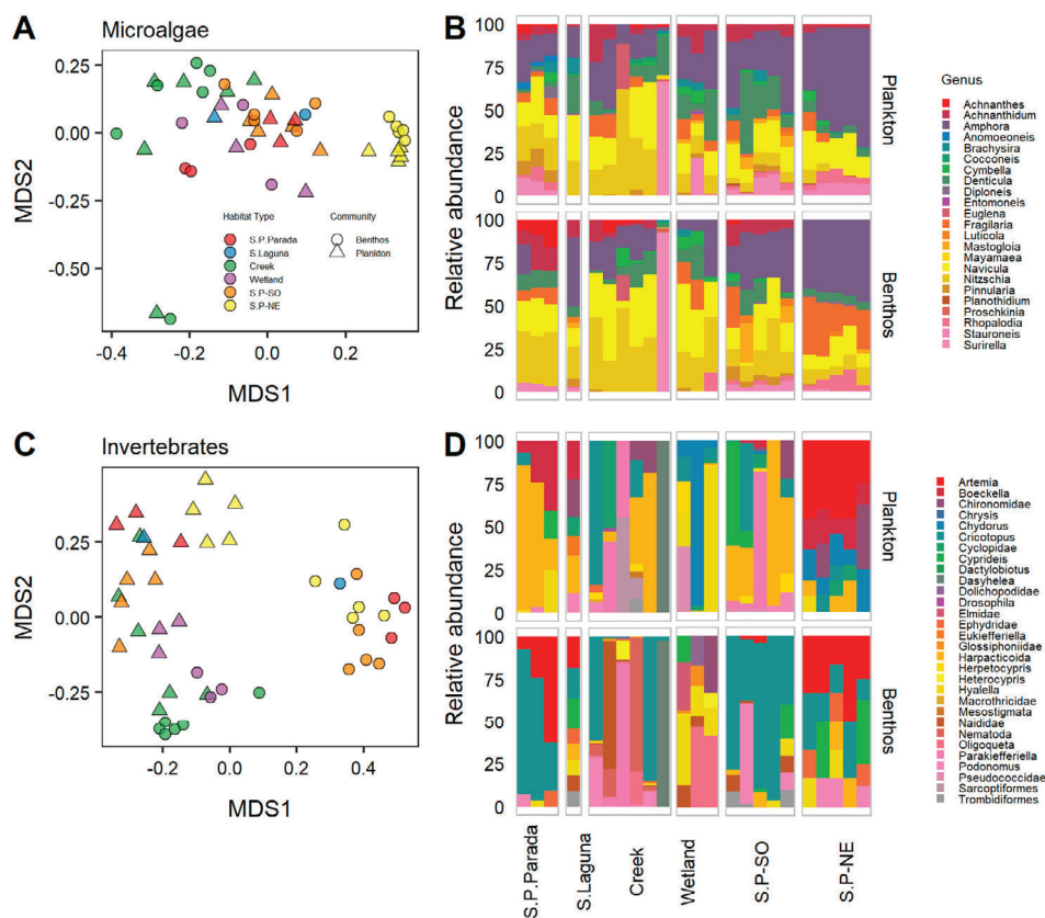
Figure 4. Beta diversity of microalgae (A), invertebrates (C) of Salar de Pedernales Basin. Relative abundances of microalgae (B) and invertebrates (D). Beta diversidad de microalgas (A), invertebrados (C) de la cuenca del Salar de Pedernales. Abundancia relativa de microalgas (B) e invertebrados (D).
