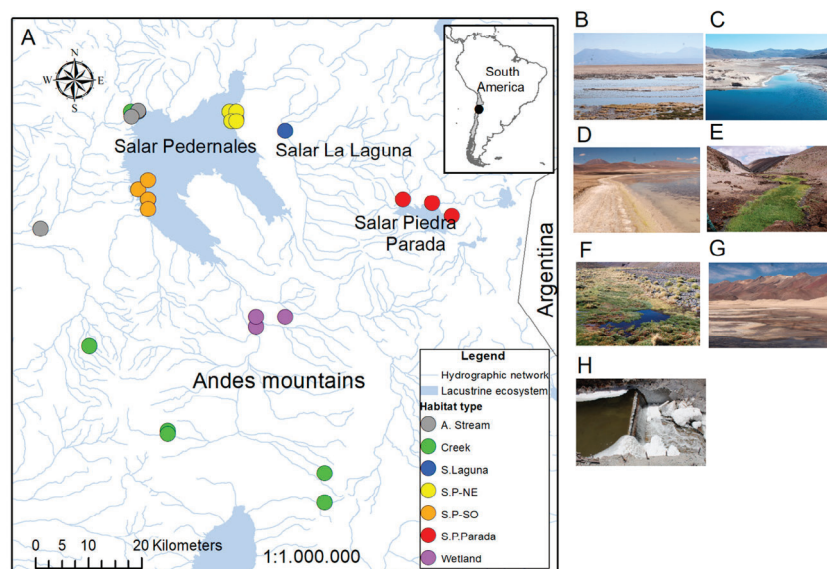
Figure 1. A) Zone of study. Salar Pedernales Basin and habitat types (B-H). B) Salar Pedernales SO, C) Salar Pedernales NE, D) Salar La Laguna, E) Creek, F) Wetland, G) Salar Piedra Parada, and H) Artificial stream. A) Zona de estudio. Cuenca del Salar de Pedernales y tipos de habitats (B-H). B) Salar Pedernales SO, C) Salar Pedernales NE, D) Salar La Laguna, E) Arroyo, F) Humedal, G) Salar Piedra Parada, y H) Canal artificial.
