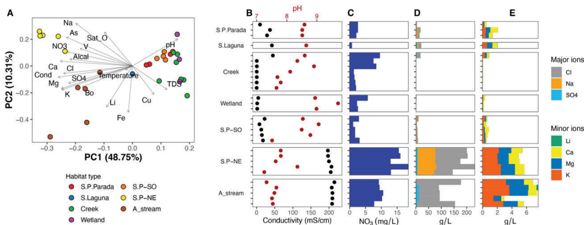
Figure 2. Environmental variables of Salar Pedernales Basin and main contributors to brine variability. A) Principal components analysis (PCA) with the habitat type, B) Conductivity and pH, C) \text{NO}_3^- concentration, D) major ( \text{Cl}^- , \text{Na}^+ and \text{SO}_4^{2-} ) and E) minor ions ( \text{Li}^+ , \text{Ca}^{2+} , \text{Mg}^{2+} and \text{K}^+ ). Variables ambientales de la cuenca del Salar de Pedernales y principales contribuyentes a la variabilidad de la salmuera. A) Análisis de componentes principales (PCA) con el tipo de hábitat, B) Conductividad y pH, C) Concentración de \text{NO}_3^- , D) Iones mayores ( \text{Cl}^- , \text{Na}^+ y \text{SO}_4^{2-} ) y E) menores ( \text{Li}^+ , \text{Ca}^{2+} , \text{Mg}^{2+} y \text{K}^+ ).
