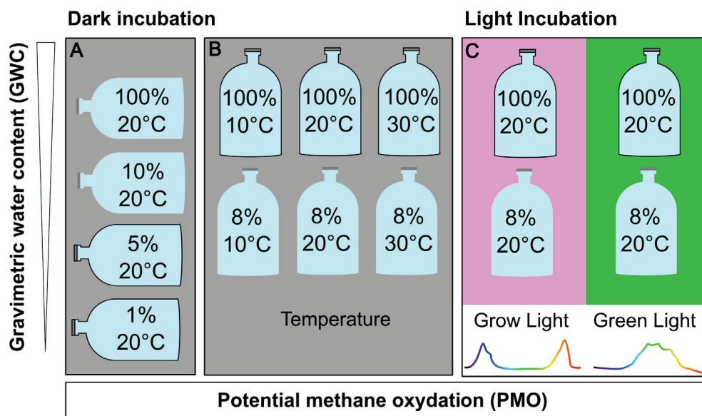
Figure 1. Overview of the experimental setup. The sediment incubation treatments included dark incubations with a gradient of gravimetric water content (GWC) at constant temperature (A), dark incubations of wet and dry sediment over a gradient of temperatures (B), as well as light incubation at constant temperature with both plant grow (photosynthesis promoting) light and green (photosynthesis-limiting) green light (C). All incubations were performed in four replicate vials except for treatment B at 10°C (three replicates). Note that the spectral distribution of the light sources is provided in an exemplary fashion (see SI Fig. 2 for details). Visión general del diseño experimental. Los tratamientos incluyeron incubaciones oscuras con un gradiente de contenido gravimétrico de agua (GWC) a temperatura constante (A), incubaciones oscuras de sedimento saturado de agua y seco sobre un gradiente de temperaturas (B), así como incubación con luz a temperatura constante tanto con luz de crecimiento vegetal (promotora de la fotosíntesis) como con luz limitadora de la fotosíntesis (verde) (C). Todas las incubaciones se realizaron en viales (cuatro réplicas, excepto el tratamiento B a 10°C con tres réplicas). La distribución espectral de las fuentes de luz se proporciona a modo de ejemplo (SI Fig. 2 para más detalles).
