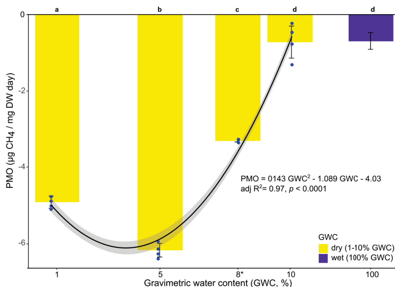
Figure 2. Potential Methane Oxidation (PMO) along a Gravimetric Water Content (GWC) gradient. Letters indicate significant differences (adjusted p < 0.05 ) between levels of GWC from post hoc following ANOVA. *Note that the values at 8% correspond to the measurements performed at 20°C for the temperature treatment. The polynomial function represents the change of PMO as a function of GWC. Oxidación potencial de metano (PMO) a lo largo de un gradiente de contenido gravimétrico de agua (GWC). Las letras indican diferencias significativas ( p ajustada < 0.05 ) entre niveles de GWC a partir de ANOVA post hoc. *Nótese que los valores al 8% corresponden a las mediciones realizadas a 20°C para el tratamiento de temperatura. La función polinómica representa el cambio de PMO en función del GWC.
