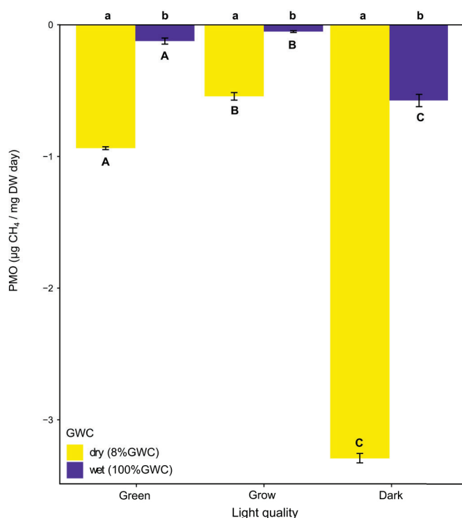
Figure 4. Potential Methane Oxidation (PMO) at three light conditions: two different light qualities (Green and Grow) with the same intensity ( 200 \mu\text{mol photon m}^{-2} \text{s}^{-1} ) and Dark conditions for sediment at 8% (dry) and 100% (wet) Gravimetric Water Content (GWC). Lower case letters indicate significant differences (adjusted p < 0.05 ) within light quality levels from post hoc following ANOVA. Upper case letters indicate significant differences (adjusted p < 0.05 ) within GWC among light qualities from post hoc following ANOVA. Oxidación Potencial de Metano (PMO) en tres calidades de luz: dos calidades diferentes (Verde y Crecimiento) con la misma intensidad ( 200 \mu\text{mol fotón m}^{-2} \text{s}^{-1} ) y condiciones de Oscuridad para sedimento al 8% (seco) y 100% (saturado) de Contenido Gravimétrico de Agua (GWC). Las letras minúsculas indican diferencias significativas ( p ajustada < 0.05 ) dentro de los niveles de calidad de la luz a partir del ANOVA post hoc siguiente. Las letras mayúsculas indican diferencias significativas ( p ajustada < 0.05 ) dentro del GWC entre calidades de luz a partir de ANOVA post hoc.
