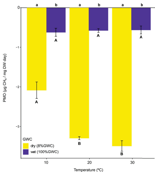
Figure 3. Potential Methane Oxidation (PMO) along a temperature gradient for sediment at 8% (dry) and 100% (wet) Gravimetric Water Content (GWC). Lower case letters indicate significant differences (adjusted p < 0.05 ) within temperature levels from post hoc following ANOVA. Upper case letters indicate significant differences ( p < 0.05 ) within GWC among temperatures following ANOVA. Oxidación Potencial de Metano (PMO) a lo largo de un gradiente de temperatura para sedimentos al 8% (seco) y 100% (saturado) de Contenido Gravimétrico de Agua (GWC). Las letras minúsculas indican diferencias significativas ( p ajustada < 0.05 ) dentro de los niveles de temperatura a partir de ANOVA post hoc. Las letras mayúsculas indican diferencias significativas ( p < 0.05 ) dentro del GWC entre temperaturas tras ANOVA.
