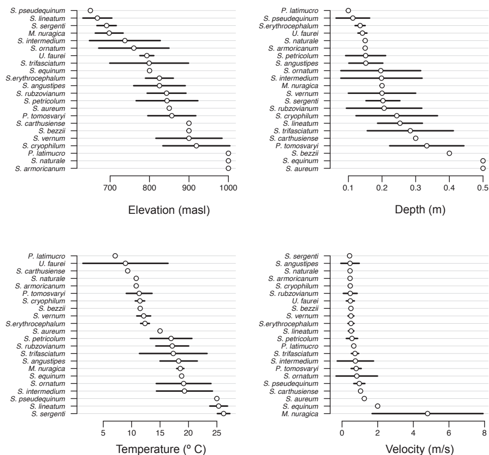
Figure 5. Optima (modes) and tolerances (error bars) for (a) elevation, (b) depth (c) temperature and (d) velocity for the mature larvae and pupae of the blackfly species found in this study. Species are arranged on the y axis by increasing optima for each variable. Óptimos y tolerancias para (a) altitud, (b) profundidad, (c) temperatura y (d) velocidad de la corriente de las larvas maduras y pupas de las especies de simúlidos identificadas en este estudio. Las especies se han ordenado en el eje y de manera ascendente según sus óptimos para cada variable.
