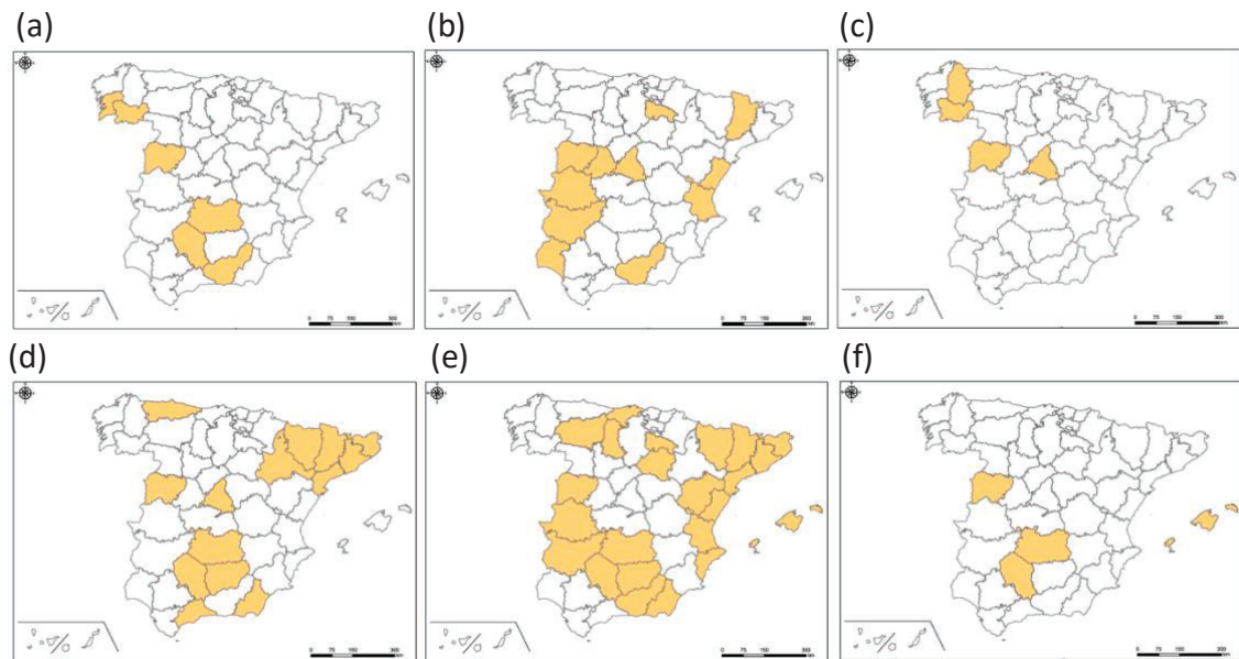
Figure 2. Provincial distribution maps for each of the six species recorded for the first time from the province of Salamanca based on this study: S. armoricanum (a), S. carthusiense (b), S. naturale (c), S. vernum (d), S. bezzii (e) and U. faurei (f). The rest of the shaded provinces indicate previous reports of these species prior to this study. Mapas de distribución provincial para cada una de las seis especies registradas por primera vez en la provincia de Salamanca basado en este estudio: S. armoricanum (a), S. carthusiense (b), S. naturale (c), S. vernum (d), S. bezzii (e), and U. faurei (f). El resto de las provincias sombreadas indican registros previos de estas especies antes de este estudio.
