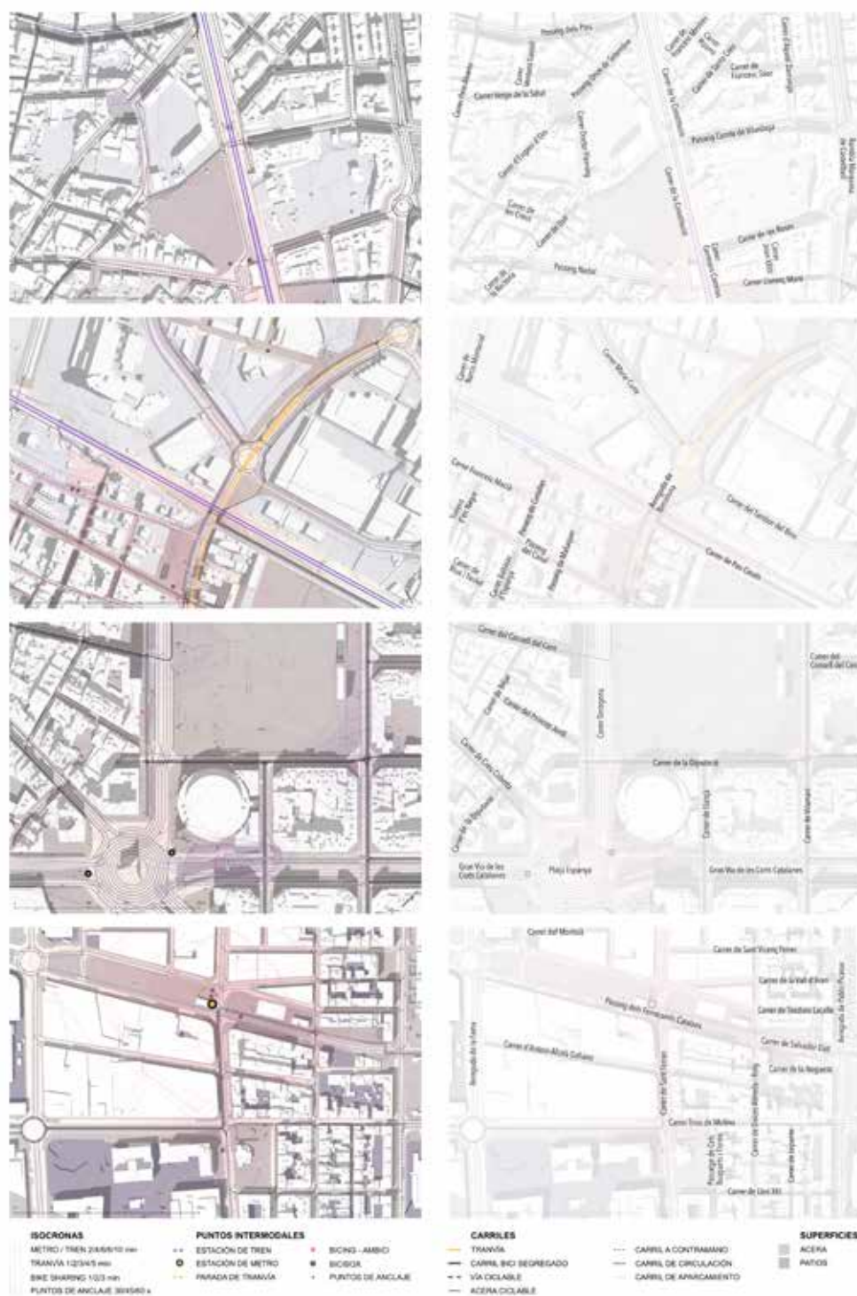
FIG. 5 / Planos de detalle de la infraestructura ciclable en diferentes contextos metropolitanos de Barcelona y esquema básico de nomenclátor viario. De arriba a abajo, Can Nadal en Sant Feliu de Llobregat, Fontsanta en Sant Joan Despí, Eixample en Barcelona y Almena en Cornellà de Llobregat
