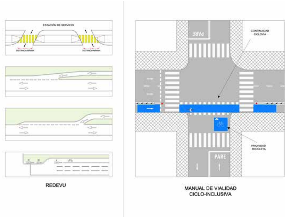
FIG. 4 / Soluciones viales propuestas para un acceso a una estación de servicio y el encuentro de una ciclovía con una calle por parte de las Recomendaciones para el Diseño de Elementos de Infraestructura Vial Urbana, REDEVU (izquierda), y de una intersección de dos calles por parte del manual de Vialidad Ciclo inclusiva (derecha)
