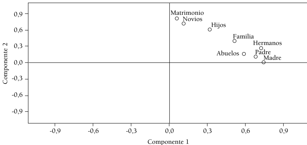
GRÁFICO 1. Gráfico de componentes en espacio rotado
