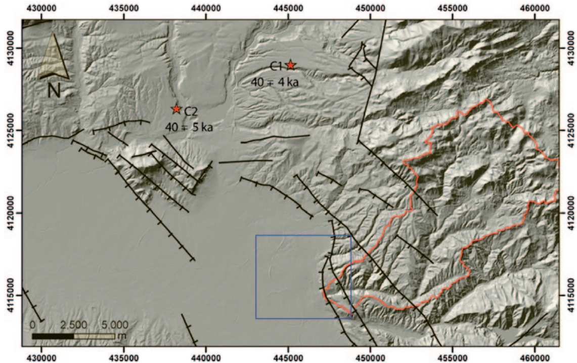
Figure 1. NW-SE normal faults outcropping in the northeastern border of the Granada basin. City of Granada is located in the blue square. C1 and C2 indicate the position of two calcretes which have been dated by U/Th radiometric method. Figura 1. Fallas normales con orientación NO-SE que afloran en el borde nororiental de la Cuenca de Granada. La ciudad de Granada está localizada en el cuadrado azul. C1 y C2 indican la localización de dos calcretes que han sido datadas mediante el método radiométrico de U/Th.
