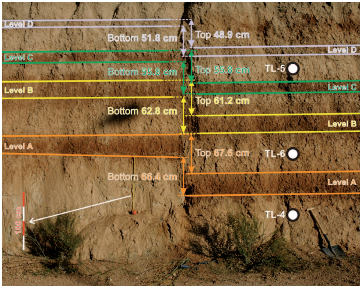
Figure 3. Paleoseismological analysis of the Granada Fault. TL-4 and TL-6 are the selected points to thermoluminescence dating. Figura 3. Análisis paleosismológico de la Falla de Granada. TL-4 y TL-6 son los puntos seleccionados para la datación mediante termoluminiscencia.
